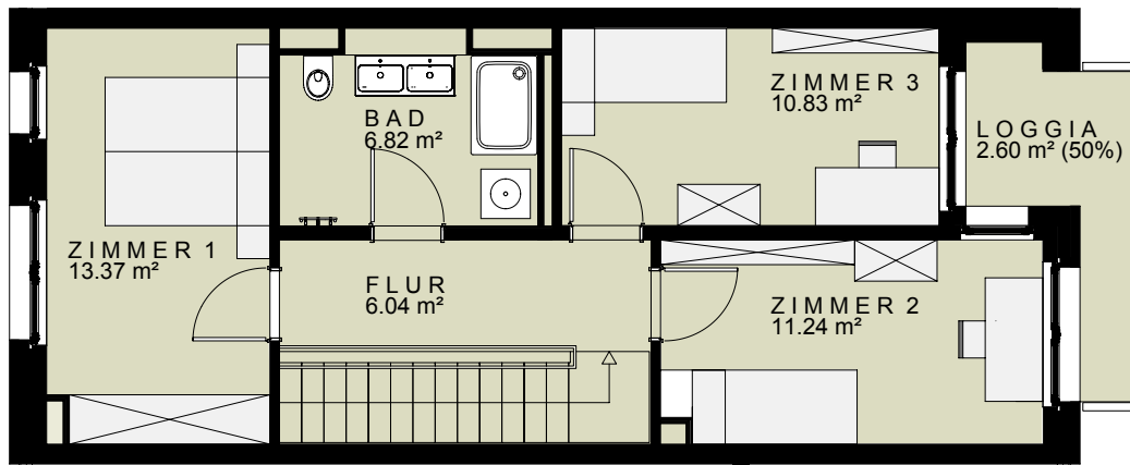
1. OBERGESCHOSS
