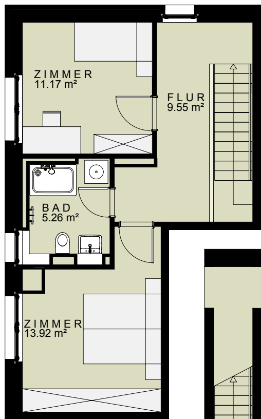
1. OBERGESCHOSS
