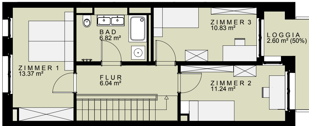
1. OBERGESCHOSS
