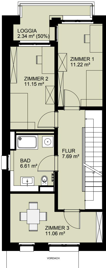
1. OBERGESCHOSS
